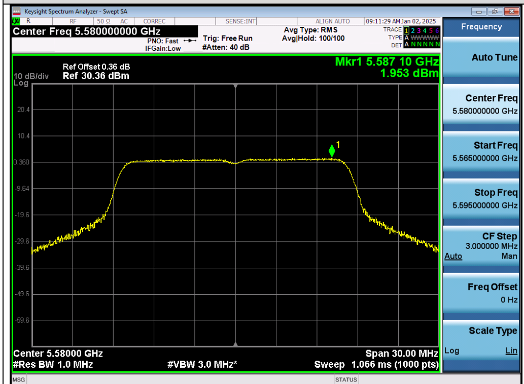
Test_Graph_802.11a_ANT1_5580_6Mbps_PSD
