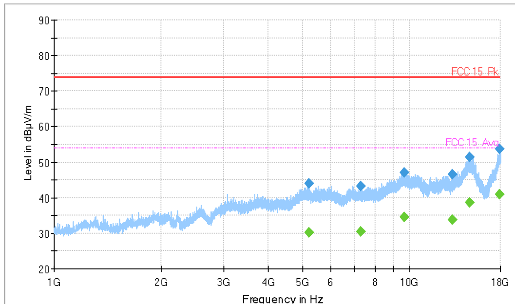
Plot 38. 1-18GHz, 1Mbps, 2402MHz
