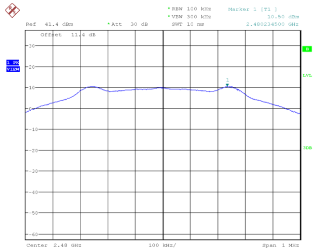
Plot 22. 2Mbps, 2480MHz Upper Band Edge
