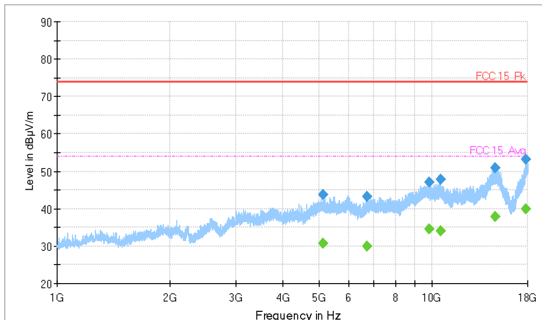
Plot 40. 1-18GHz, 1Mbps, 2480MHz
