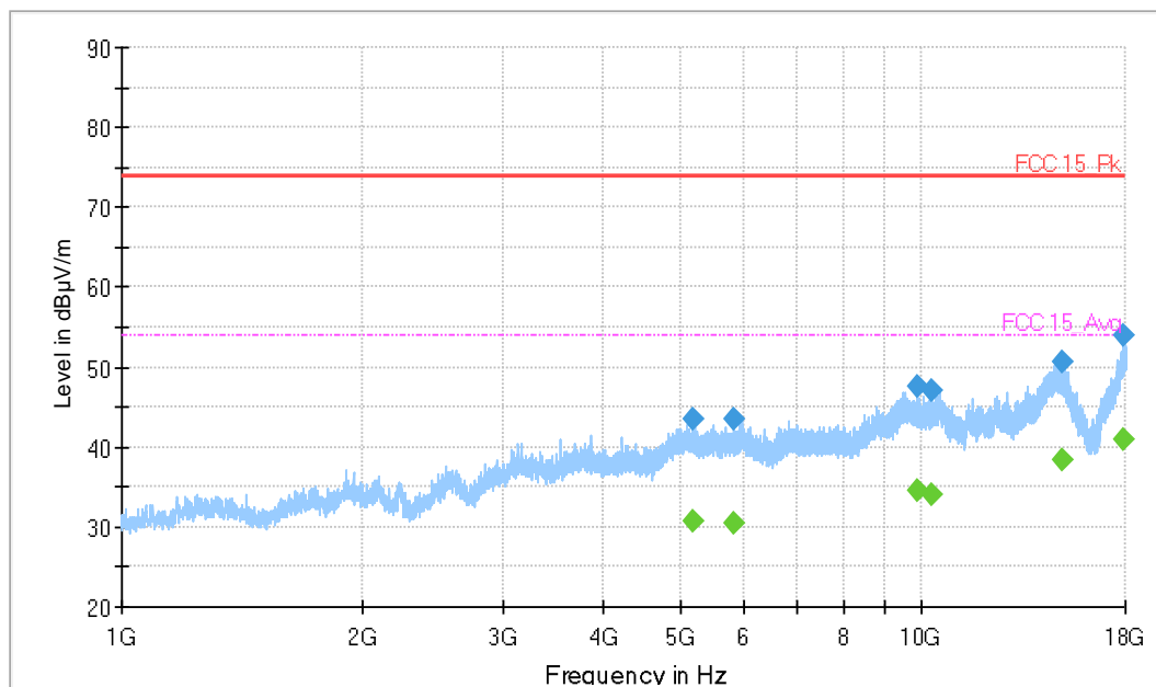
Plot 39. 1-18GHz, 1Mbps, 2440MHz
