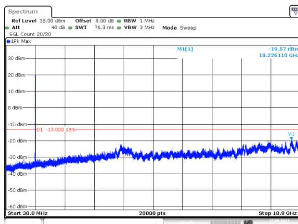
5MHz_Middle_QPSK_25@0
