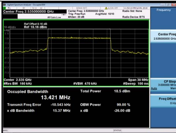
MCH_QPSK_75RB#0
