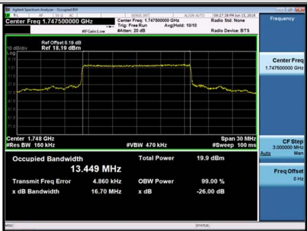
HCH_QPSK_75RB#0
