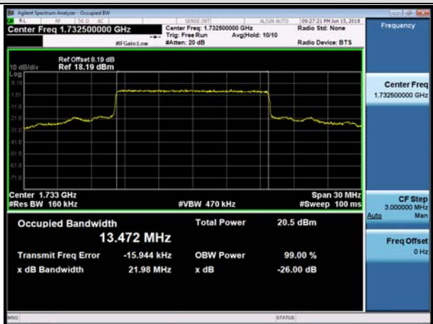
MCH_QPSK_75RB#0
