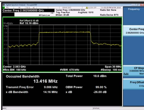
HCH_QPSK_75RB#0
