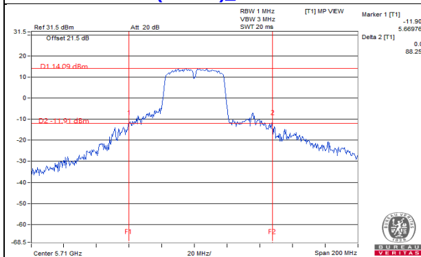
802.11ac (VHT40)_Chain 1 / CH142
