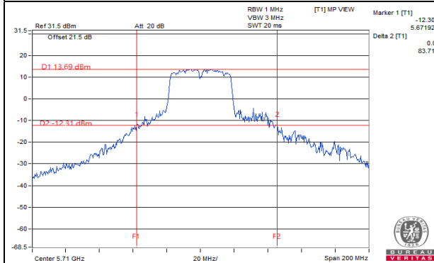
802.11ac (VHT40)_Chain 1 / CH142
