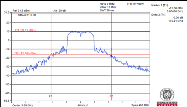
802.11ac (VHT80)_Chain 1 / CH138
