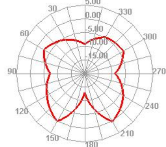
2450.000MHz E2
