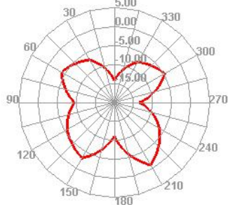
2400.000MHz E1
