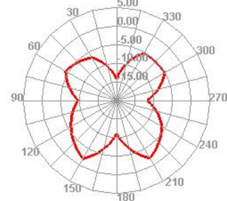
2400.000MHz E2
