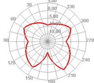
2450.000MHz E1
