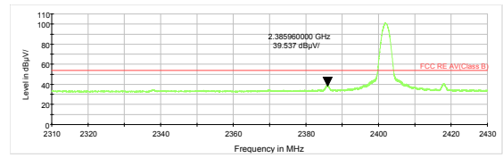
BLE Channel 0 Average
