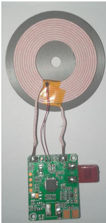
PCBA Top
