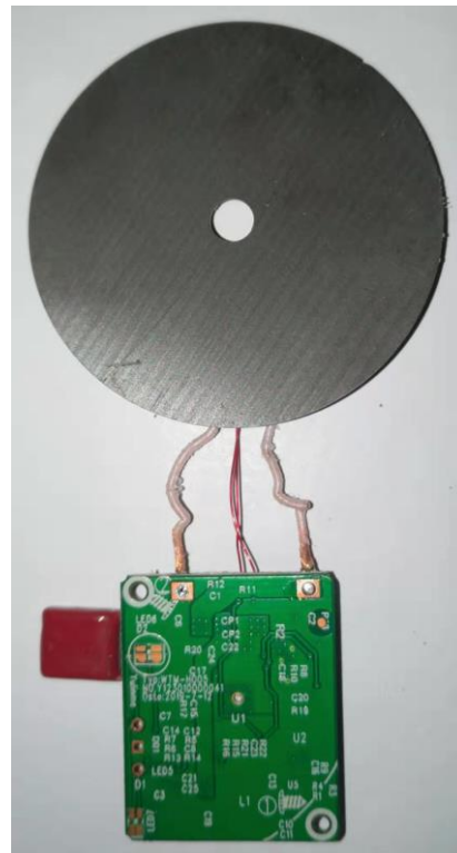
PCBA Bottom
