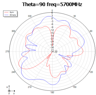
Theta=90 freq=5700MHz
