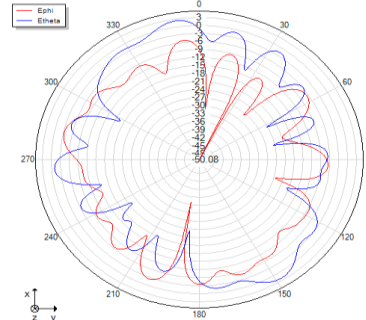
Theta=90 freq=5700MHz
