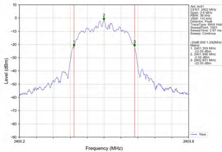
Pi/4DQPSK 2DH5 LCH 2402MHz Ant1 NTN
