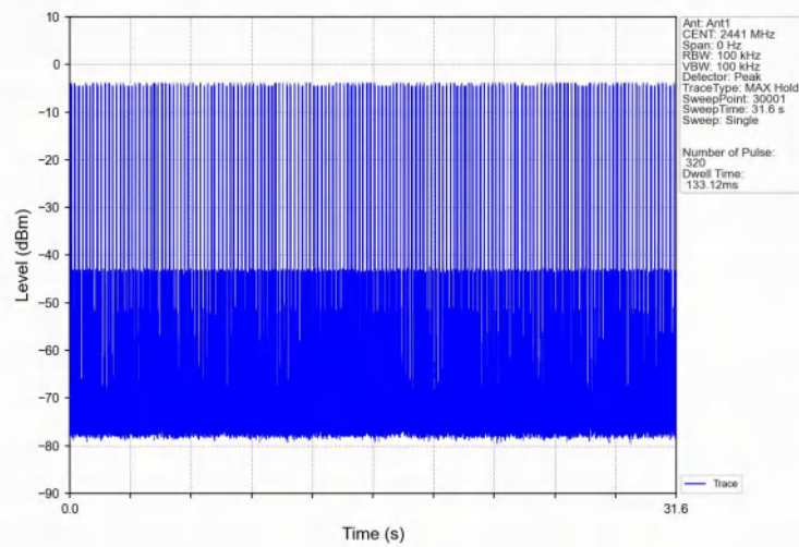
8DPSK_3DH1_HOPP_Ant1_NTNV
