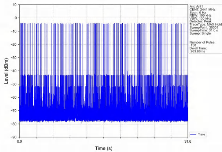
8DPSK_3DH3_HOPP_Ant1_NTNV
