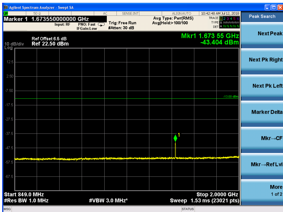
Channel 384, 849MHz~2GHz
