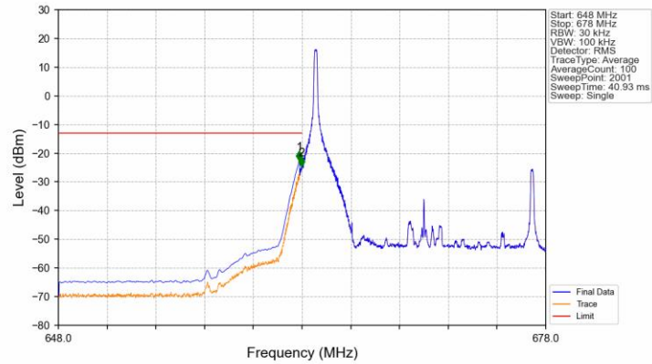
Band71_15MHz_QPSK_LCH_670.5MHz_RB_1_0_NTNV
