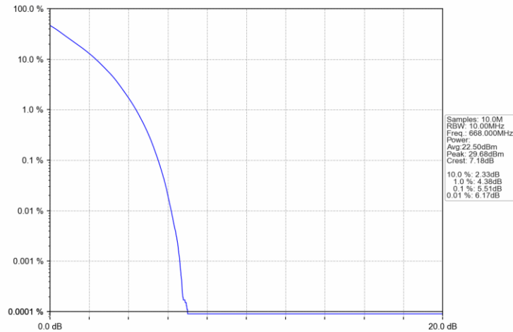
Band71_10MHz_QPSK_LCH_668MHz_RB_50_0_NTNV
