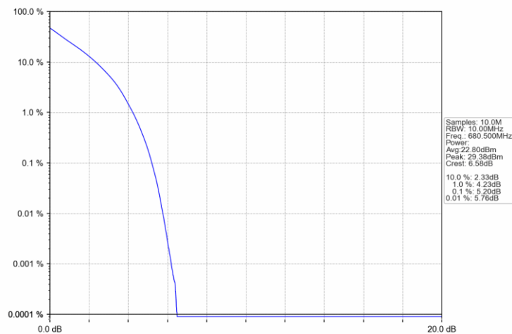
Band71_10MHz_QPSK_MCH_680.5MHz_RB_50_0_NTNV
