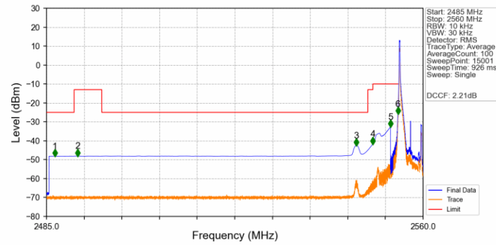
Band41_5MHz_QPSK_LCH_2557.5MHz_RB_1_0_NTNV
