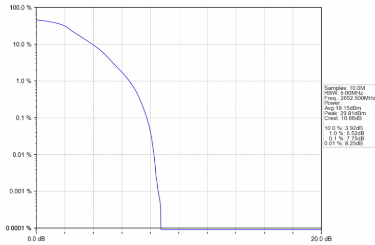
Band41_5MHz_QPSK_HCH_2652.5MHz_RB_25_0_NTNV
