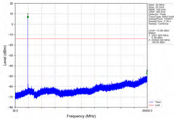
GFSK DH5 LCH 2402MHz_Ant1_NTNV
