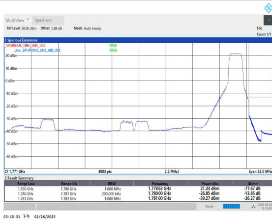
Band66_20MHz_QPSK_132572_1RB#99
