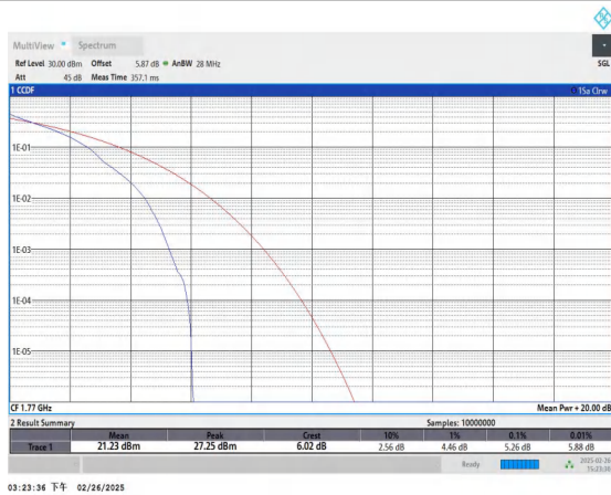
Band66-20MHz-QPSK-132572-1RB#0-PASS
