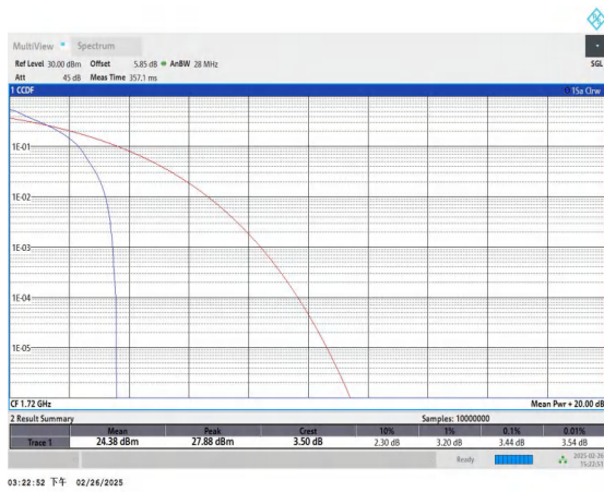
Band66-20MHz-QPSK-132072-1RB#0-PASS
