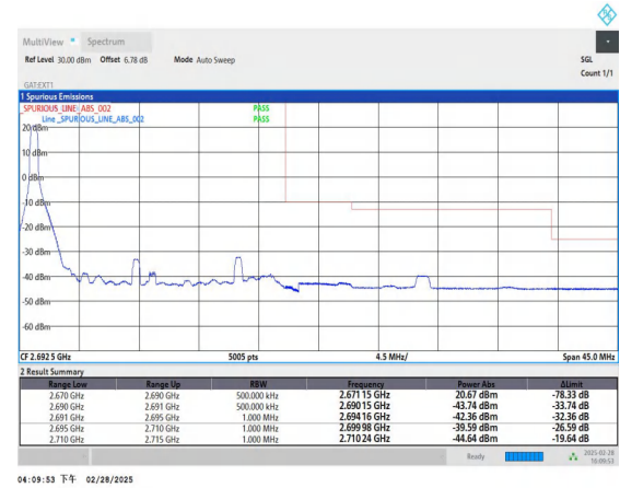
Band41_20MHz_QPSK_41490_1RB#0
