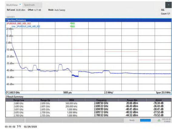
Band41_10MHz_QPSK_41540_1RB#0
