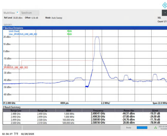
Band41_10MHz_QPSK_39740_1RB#0
