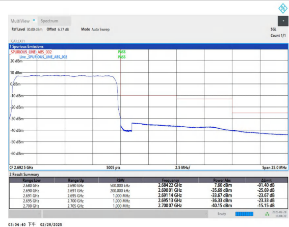
Band41_10MHz_QPSK_41540_50RB#0
