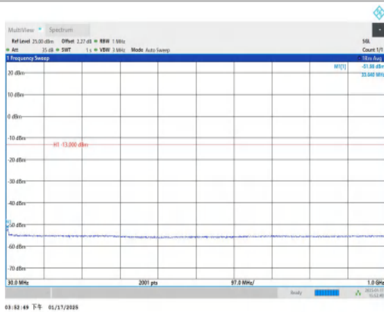
Band4-1513-30~1000MHz-PASS
