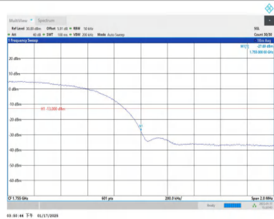
Band4-1513-PASS
