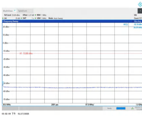
Band4-1413-30~1000MHz-PASS
