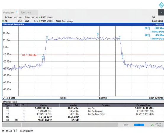
Band4-10MHz-QPSK-20000-50RB#0-PASS
