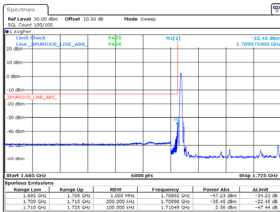
n66_15MHz_15kHz_1717.5MHz_DFT-s-OFDM QPSK_RB1@0
