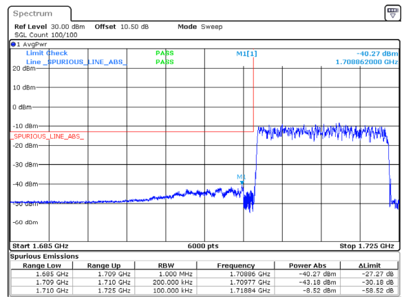
n66_15MHz_15kHz_1717.5MHz_DFT-s-OFDM QPSK_RB75@0
