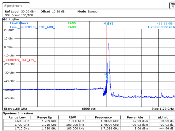
n66_20MHz_15kHz_1720MHz_DFT-s-OFDM QPSK_RB1@0
