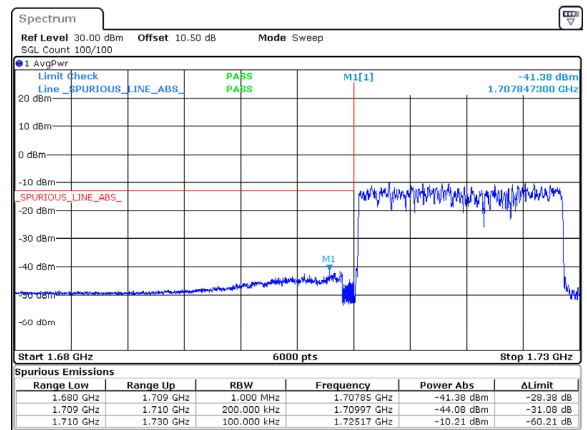
n66_20MHz_15kHz_1720MHz_DFT-s-OFDM QPSK_RB100@0
