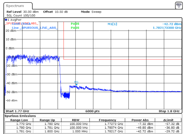
n66_10MHz_15kHz_1775MHz_DFT-s-OFDM QPSK_RB50@0
