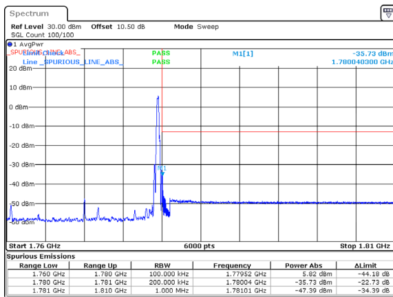
n66_20MHz_15kHz_1770MHz_DFT-s-OFDM QPSK_RB1@105
