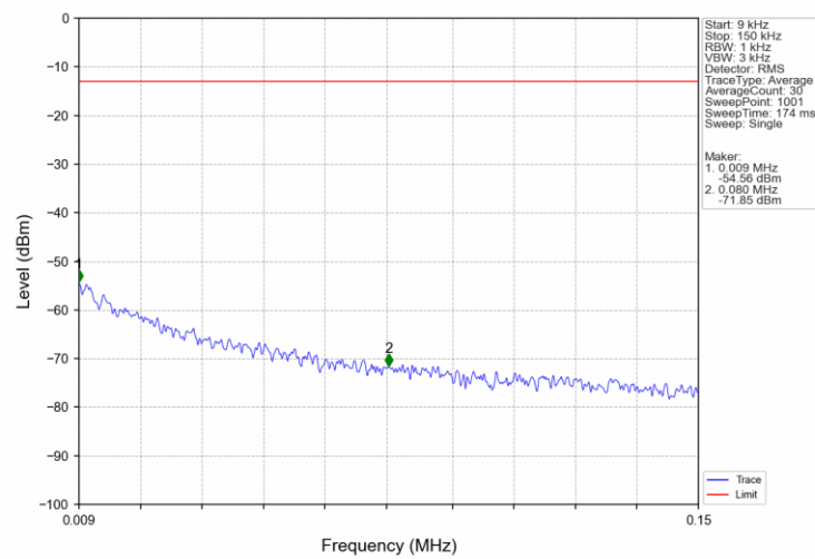
Band71_10MHz_QPSK_LCH_668MHz_RB_1_0_NTNV
