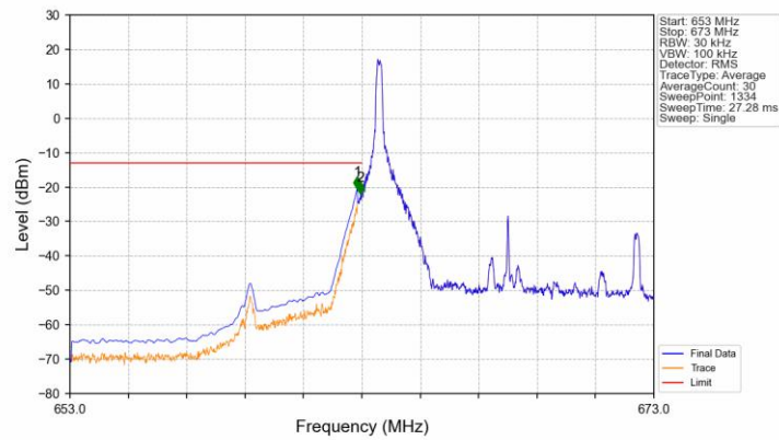
Band71_10MHz_QPSK_LCH_668MHz_RB_1_0_NTNV
