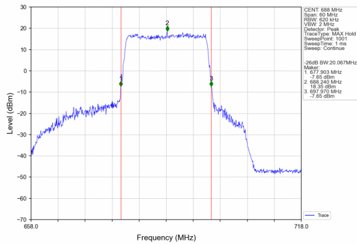
Band71_20MHz_16QAM_HCH_688MHz_RB_100_0_NTNV
