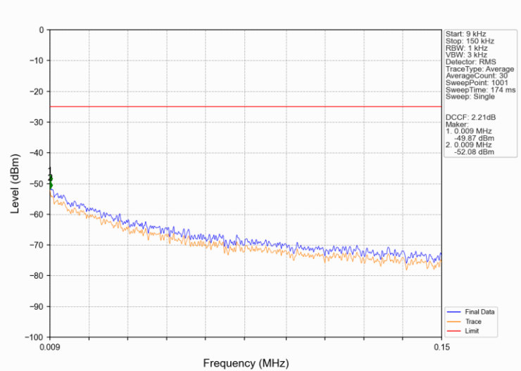
Band41 5MHz QPSK LCH 2557.5MHz RB 1 0 NTNV
