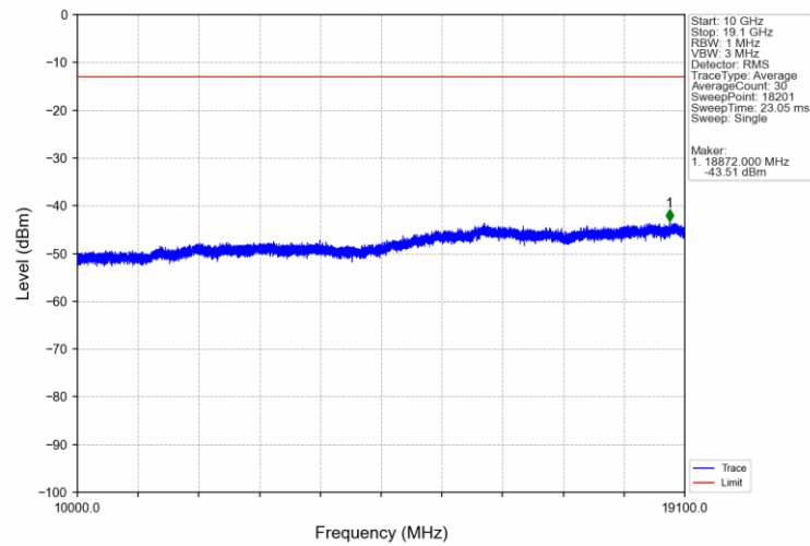
Band2_20MHz_QPSK_MCH_1880MHz_RB_1_0_NTNV
