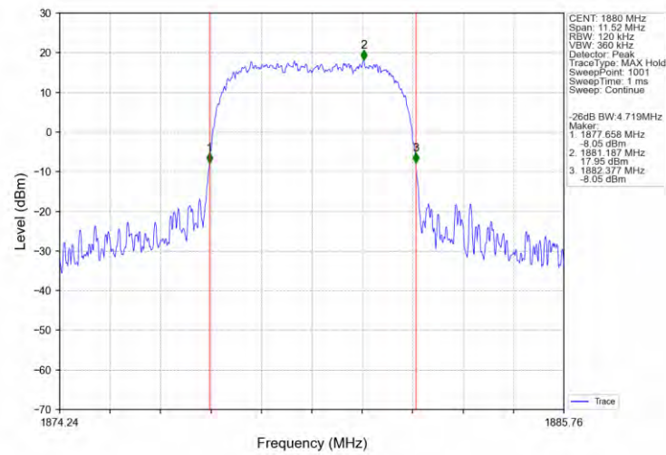
Band2_HSUPA_MCH_1880MHz_Subtest 1_NTNV
