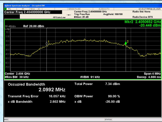
BLE 2M_Channel 1
