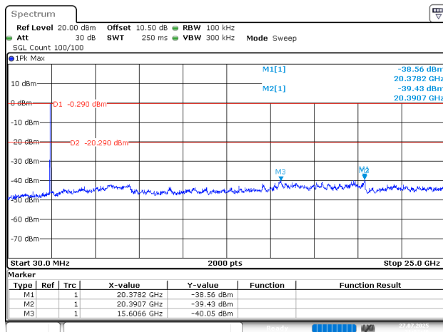
802.11g_2437MHz
