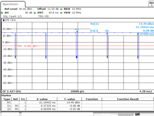
802.11b_2437MHz
