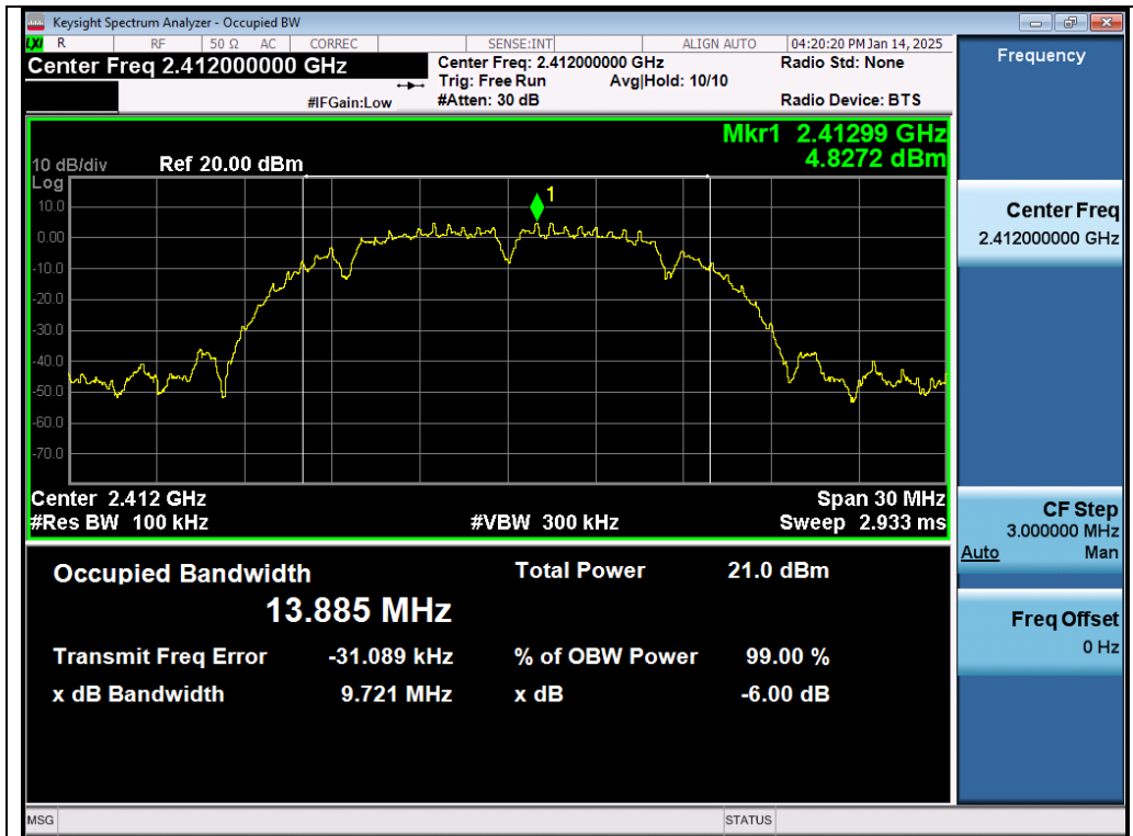
Test_Graph_802.11b_Chain A_2412_1Mbps_DTSBW
