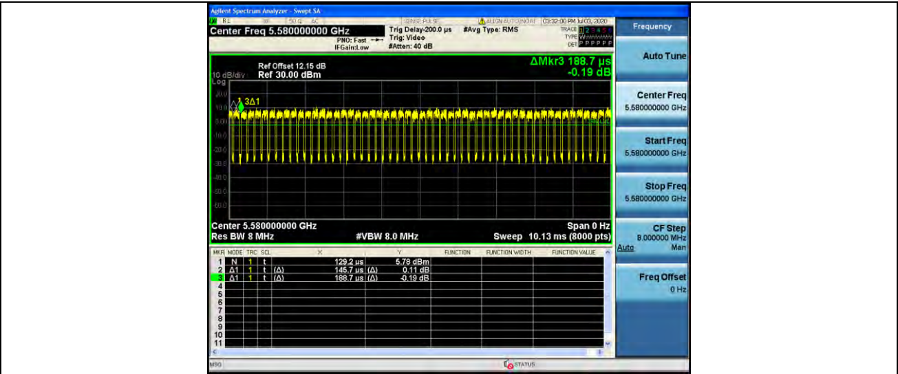
11AC20MIMO_Ant2_5580
