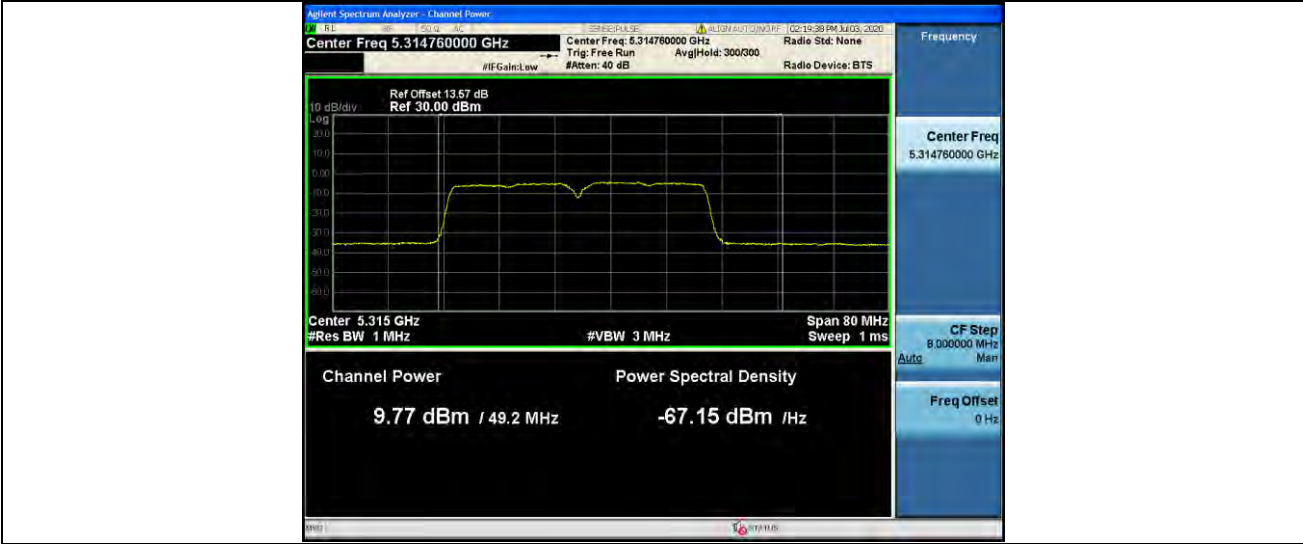
11N40MIMO_Ant2_5310
