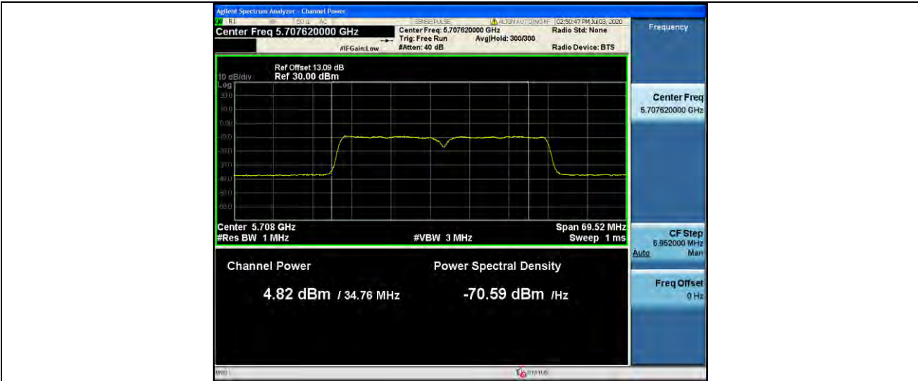
11N40MIMO_Ant2_5710_UNII-2C
