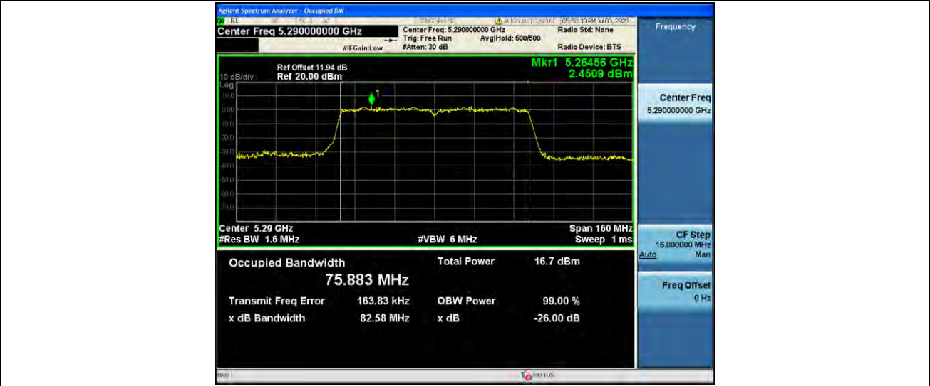
11AC80MIMO_Ant2_5290
