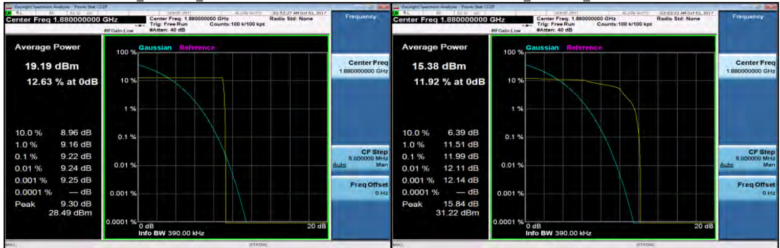
GPRS_1900MHz_MidCH661-1880
