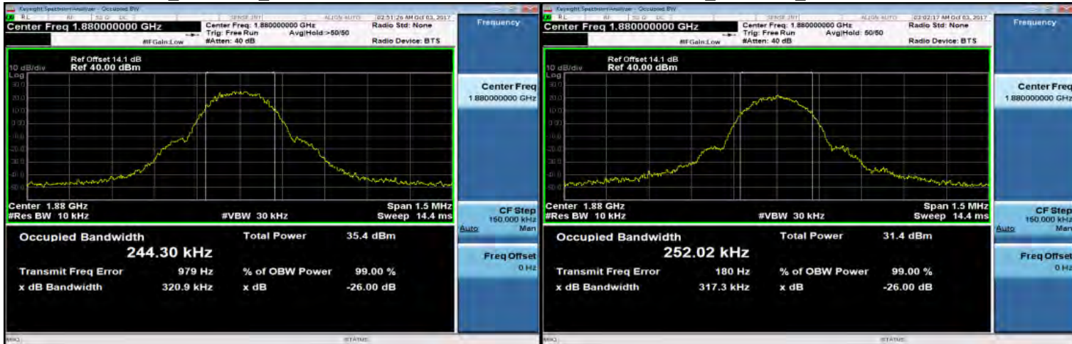
GPRS_1900MHz_MidCH661-1880
