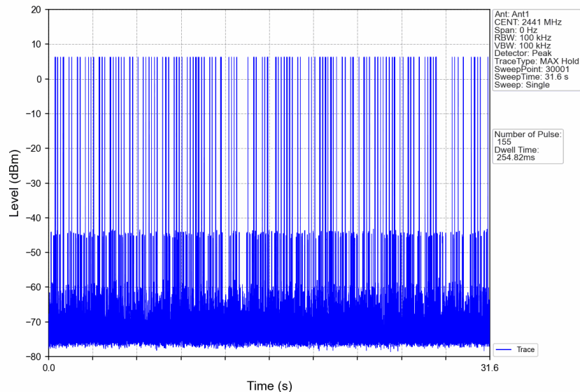
GFSK_DH3_HOPP_Ant1_NTNV
