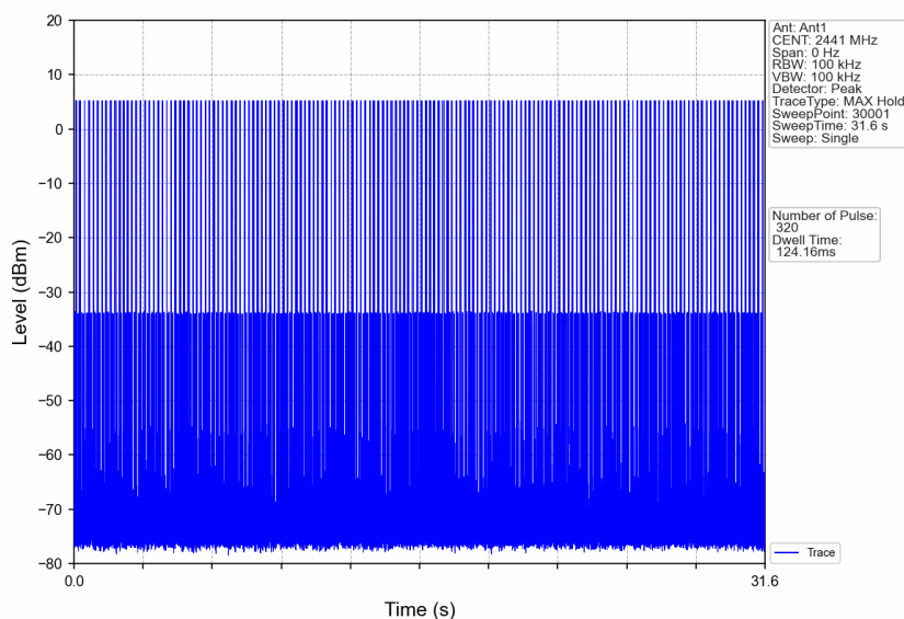
Pi/4DQPSK_2DH1_HOPP_Ant1_NTNV
