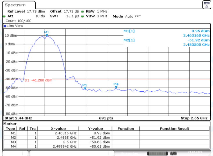
11B-Ant2-2462-PASS
