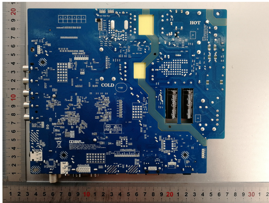
EUT – PCB-1 Module View
