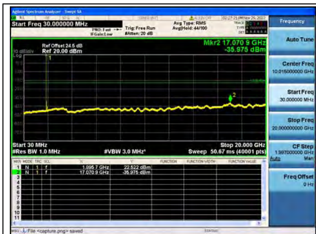
Band2 / 15MHz / High CH / QPSK
