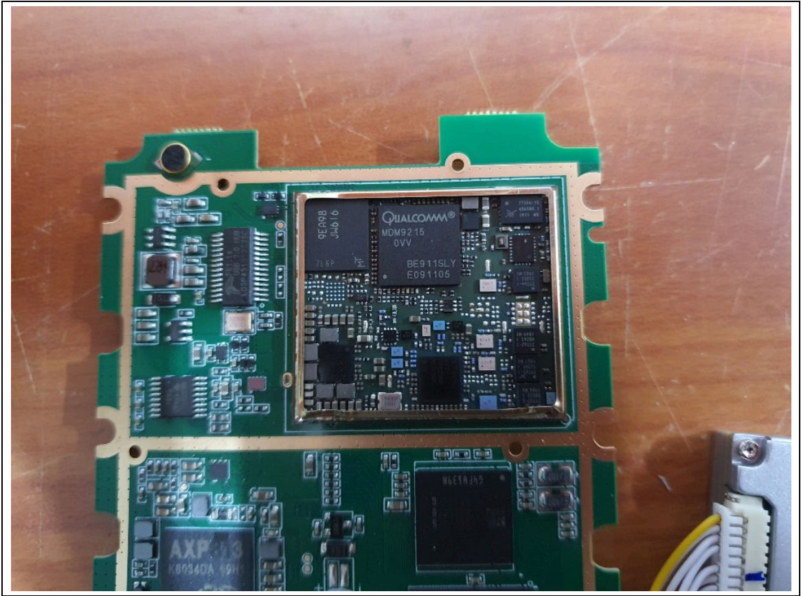
LTE Module
