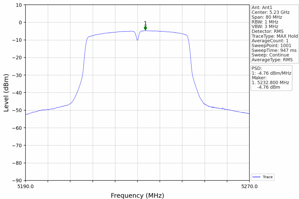
802.11n(HT40)_HCH_5230MHz_Ant1_NTNV
