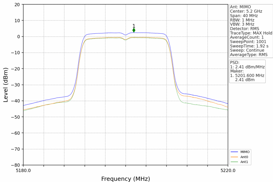
802.11n(HT20)_MCH_5200MHz_MIMO_NTNV
