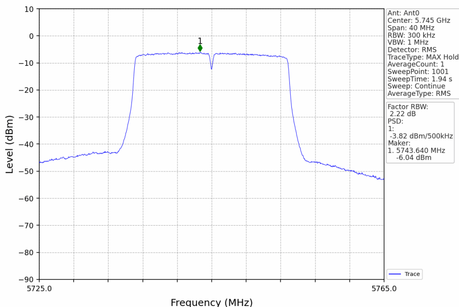
802.11ac(VHT20)_LCH_5745MHz_Ant0_NTNV
