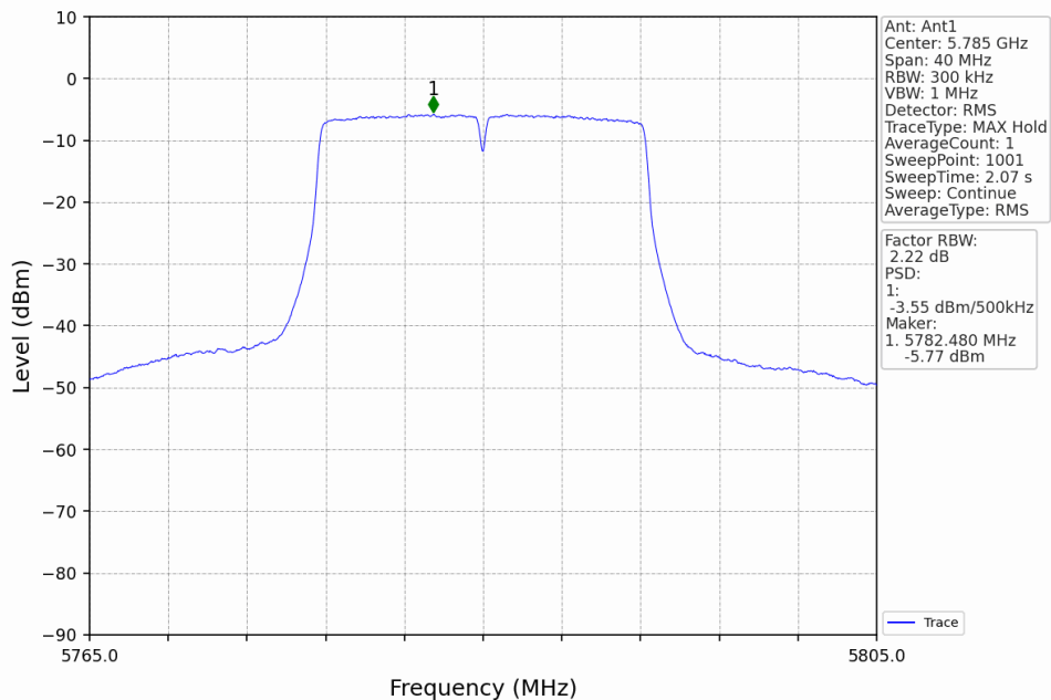
802.11a_MCH_5785MHz_Ant1_NTNV
