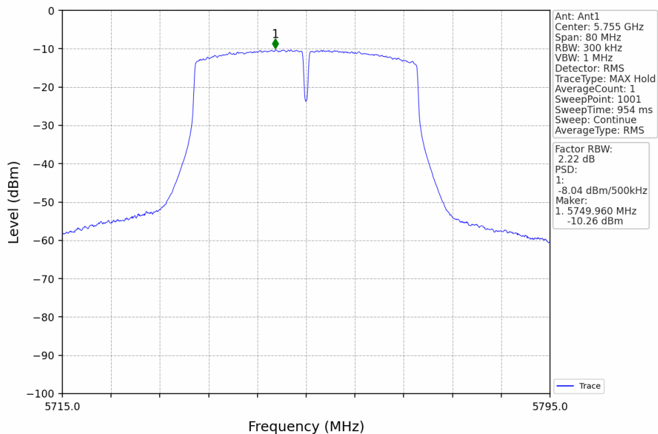
802.11ac(VHT40)_LCH_5755MHz_Ant1_NTNV
