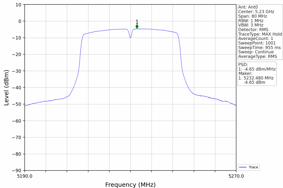
802.11ac(VHT40)_HCH_5230MHz_Ant0_NTNV
