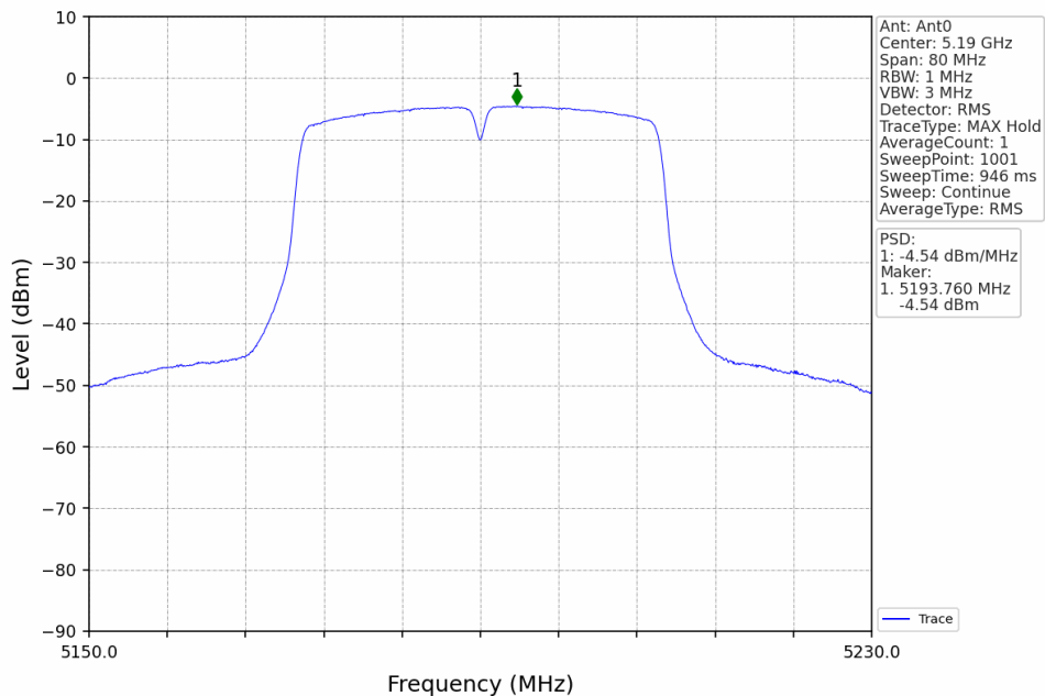
802.11n(HT40)_LCH_5190MHz_Ant0_NTNV
