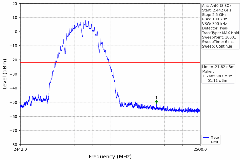
802.11b_HCH_2462MHz_Ant0 (SISO)_NTNV
