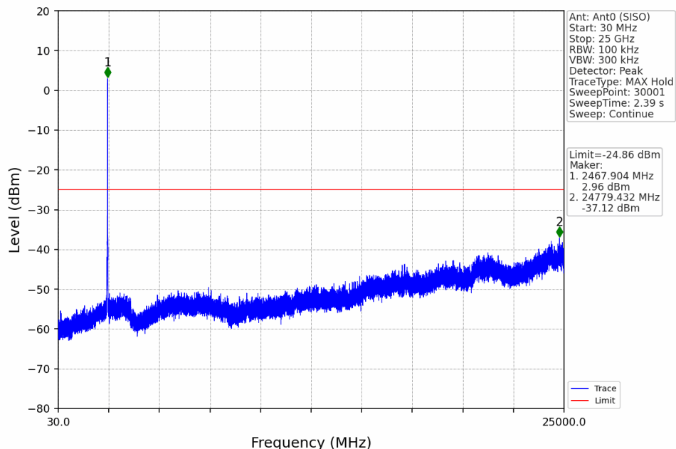
802.11g_HCH_2462MHz_Ant0 (SISO)_NTNV
