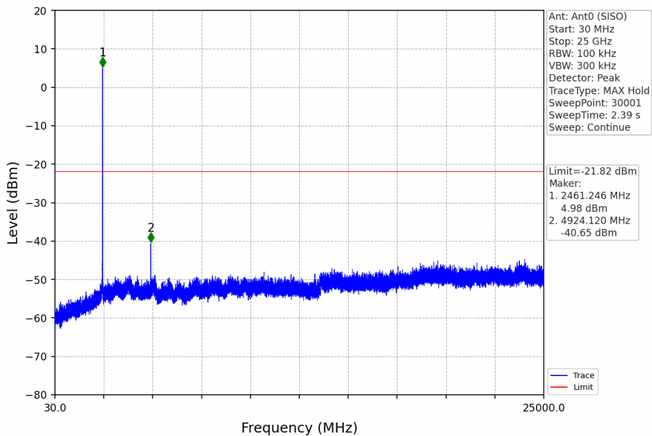
802.11b_HCH_2462MHz_Ant0 (SISO)_NTNV
