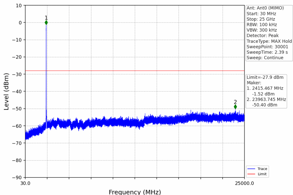
802.11n(HT20)_LCH_2412MHz_Ant0 (MIMO)_NTNV
