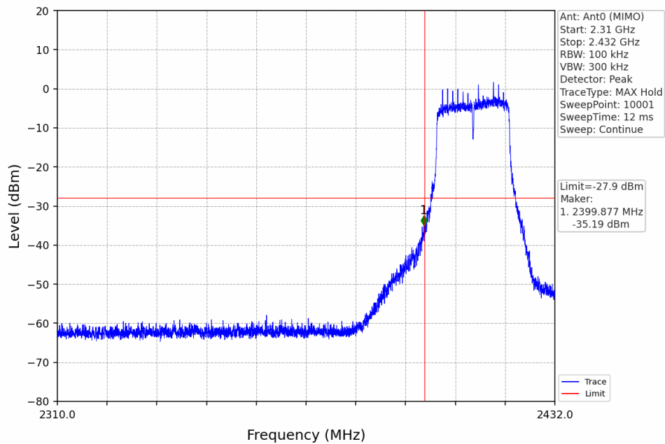
802.11n(HT20)_LCH_2412MHz_Ant0 (MIMO)_NTNV
