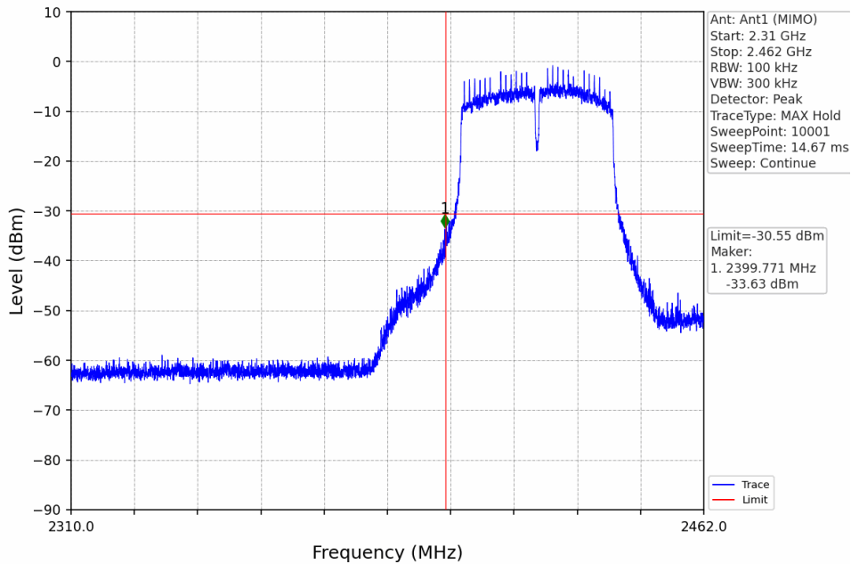
802.11n(HT40)_LCH_2422MHz_Ant1 (MIMO)_NTNV
