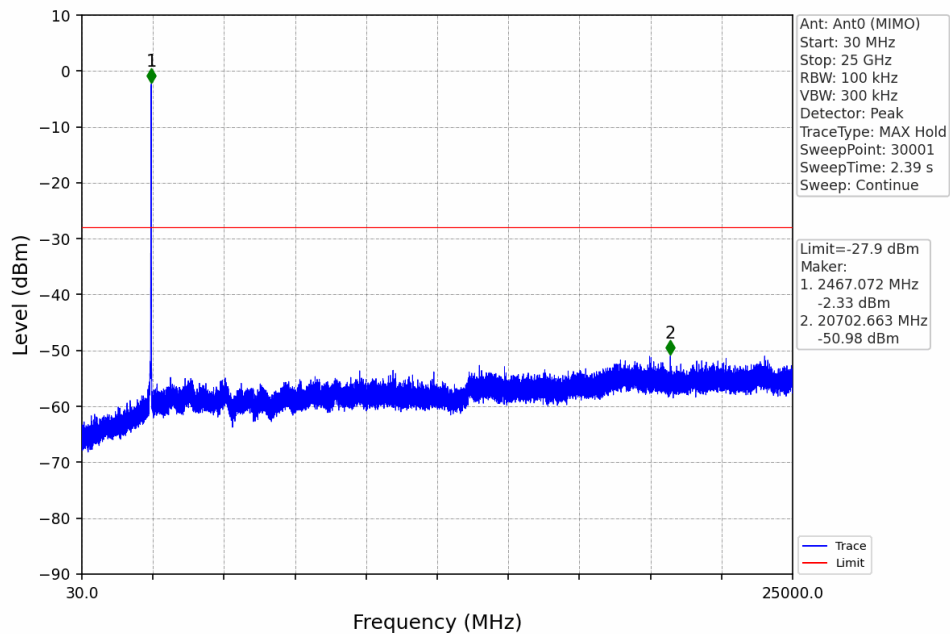
802.11n(HT20)_HCH_2462MHz_Ant0 (MIMO)_NTNV
