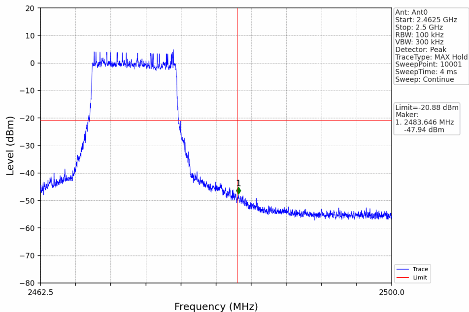
GND_10MHz_HCH_2472.5MHz_Ant0_NTNV
