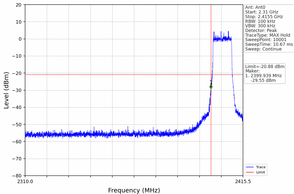
GND_10MHz_LCH_2405.5MHz_Ant0_NTNV
