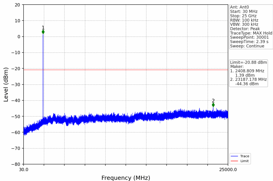
GND_10MHz_LCH_2405.5MHz_Ant0_NTNV
