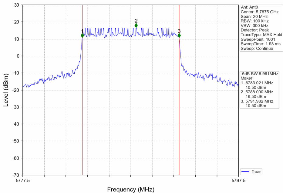
10_MCH_5787.5MHz_Ant0_NTNV
