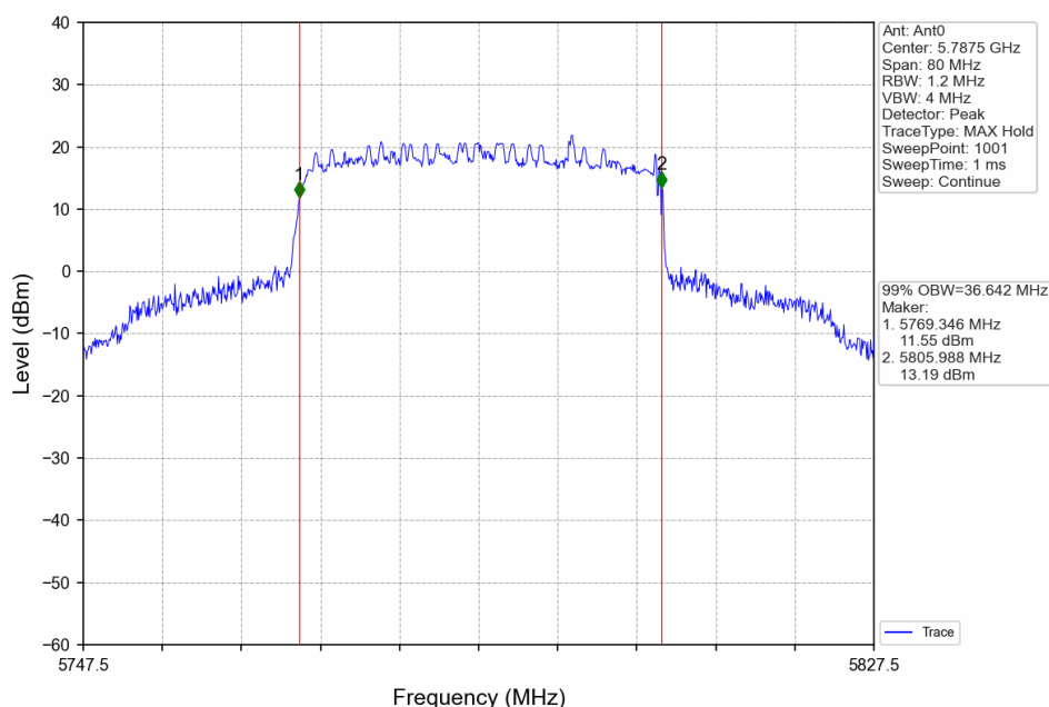
40_MCH_5787.5MHz_Ant0_NTNV
