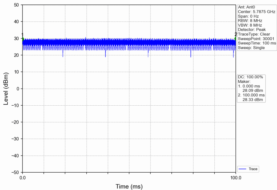
10_MCH_5787.5MHz_Ant0_NTNV
