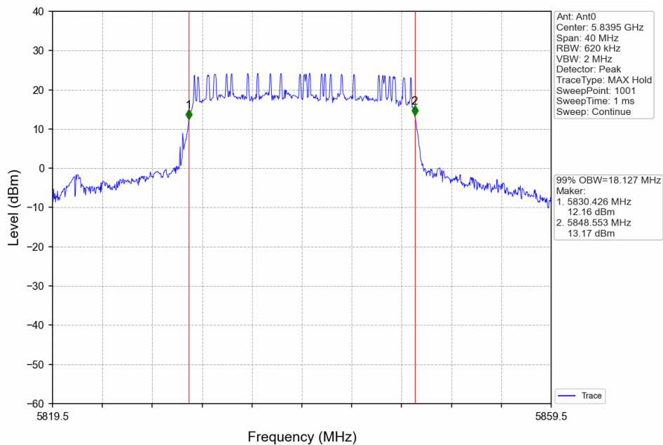
20_HCH_5839.5MHz_Ant0_NTNV
