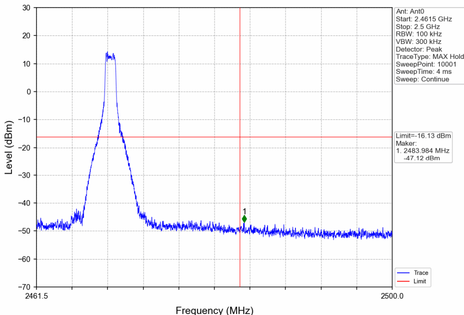
1.4M_HCH_2469.5MHz_Ant0_NTNV
