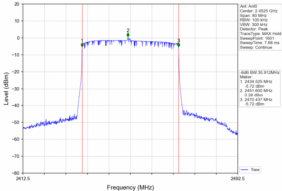
40M_HCH_2452.5MHz_Ant0_NTNV
