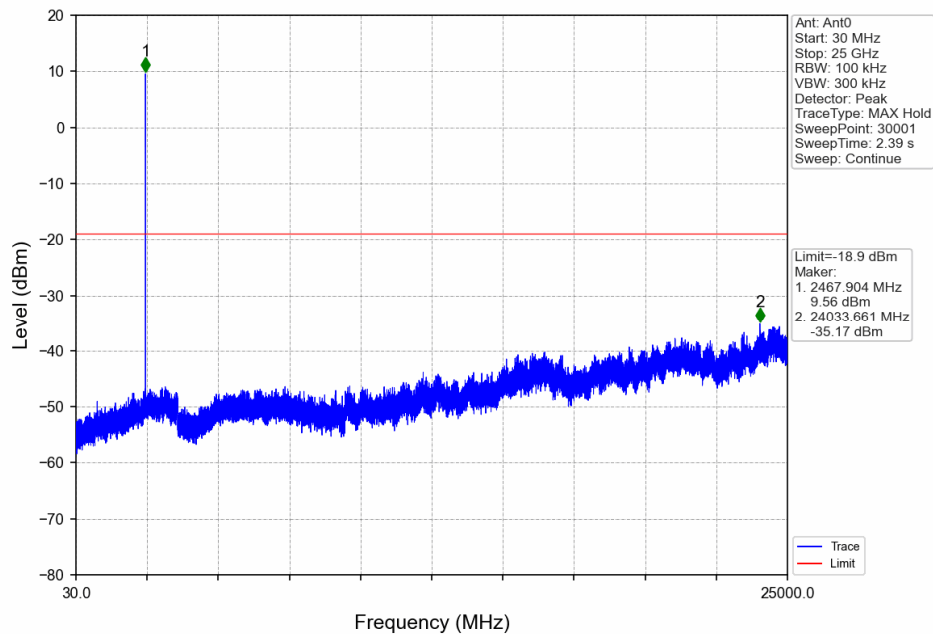
3M_HCH_2468.5MHz_Ant0_NTNV
