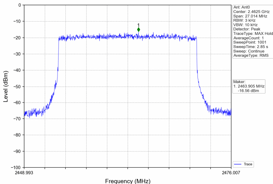
20M_HCH_2462.5MHz_Ant0_NTNV
