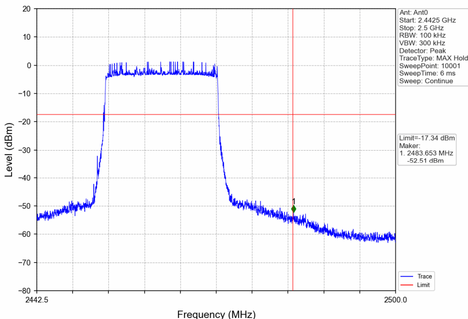
20M_HCH_2462.5MHz_Ant0_NTNV
