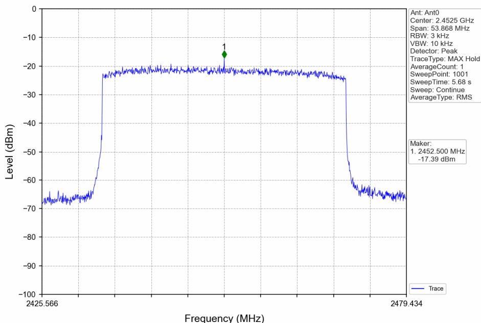
40M_HCH_2452.5MHz_Ant0_NTNV
