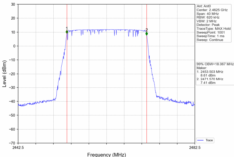
20M_HCH_2462.5MHz_Ant0_NTNV
