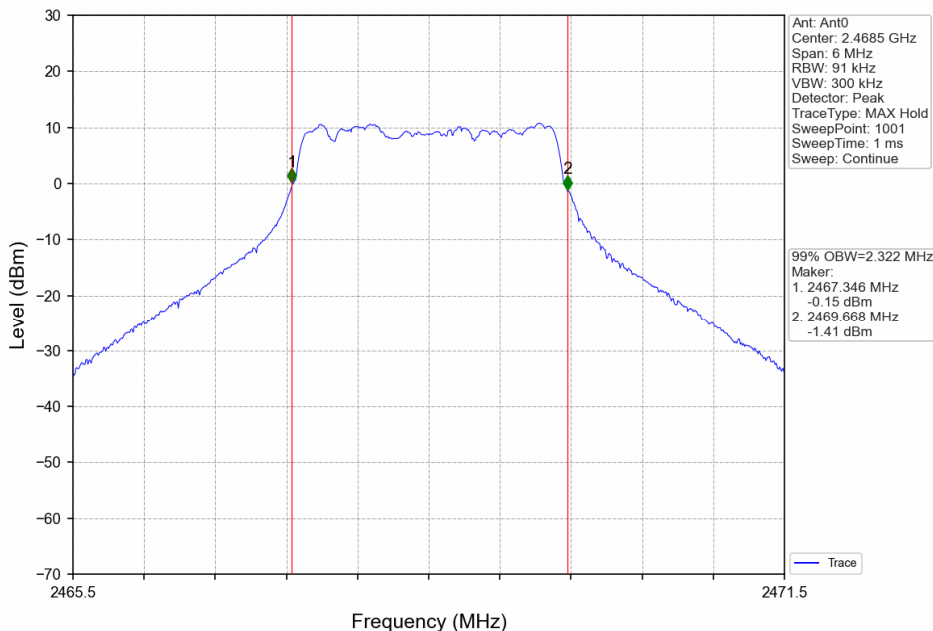
3M_HCH_2468.5MHz_Ant0_NTNV
