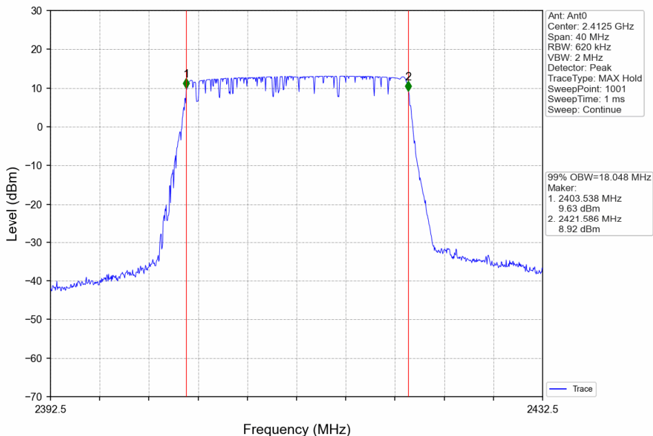
20M_LCH_2412.5MHz_Ant0_NTNV
