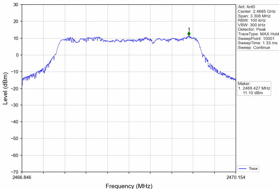
3M_HCH_2468.5MHz_Ant0_NTNV
