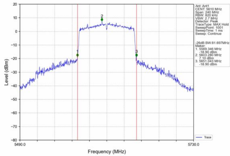
802.11ac(VHT80) HCH_5610MHz_Ant1_NTNV
