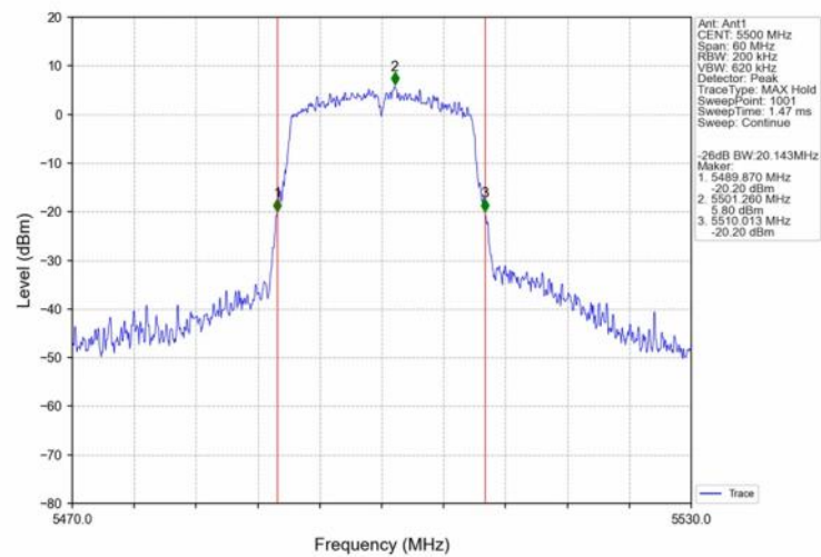
802.11n(HT20)_LCH_5500MHz_Ant1_NTNV
