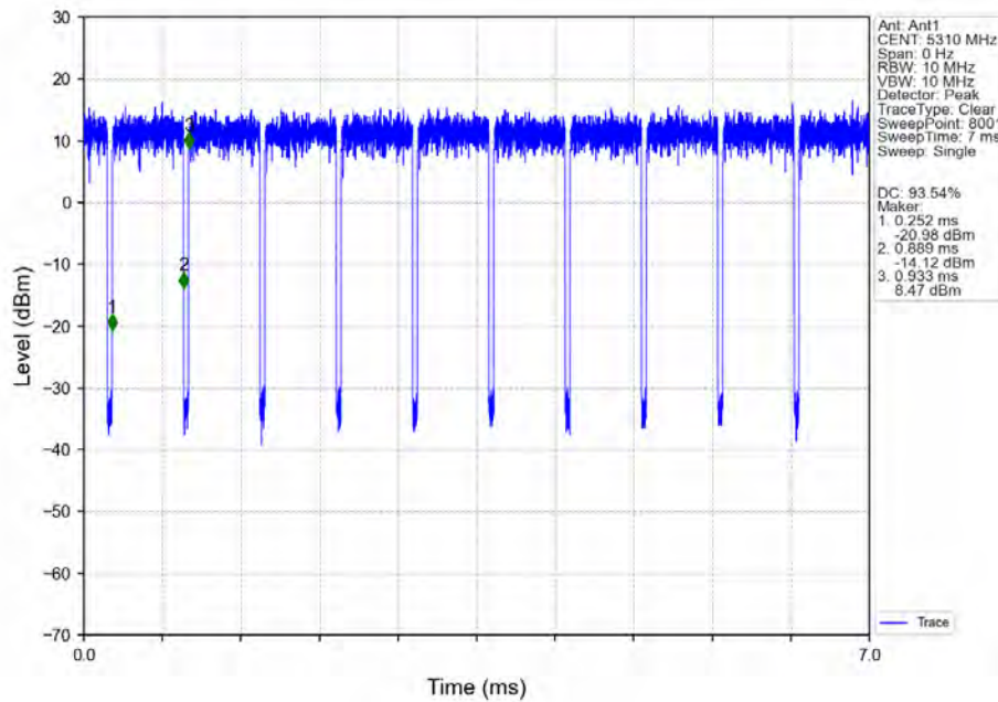
802.11n(HT40)_HCH_5310MHz_Ant1_NTNV
