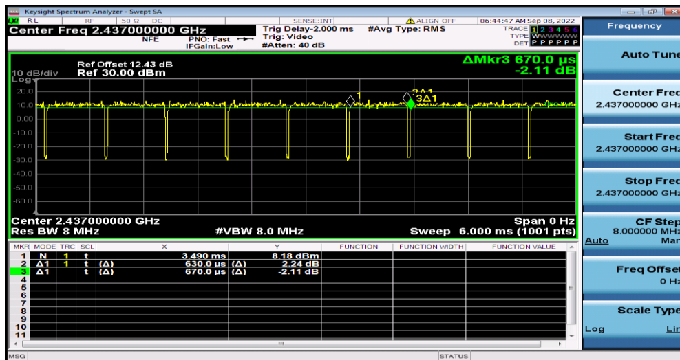
11N40MIMO_Ant2_2437
