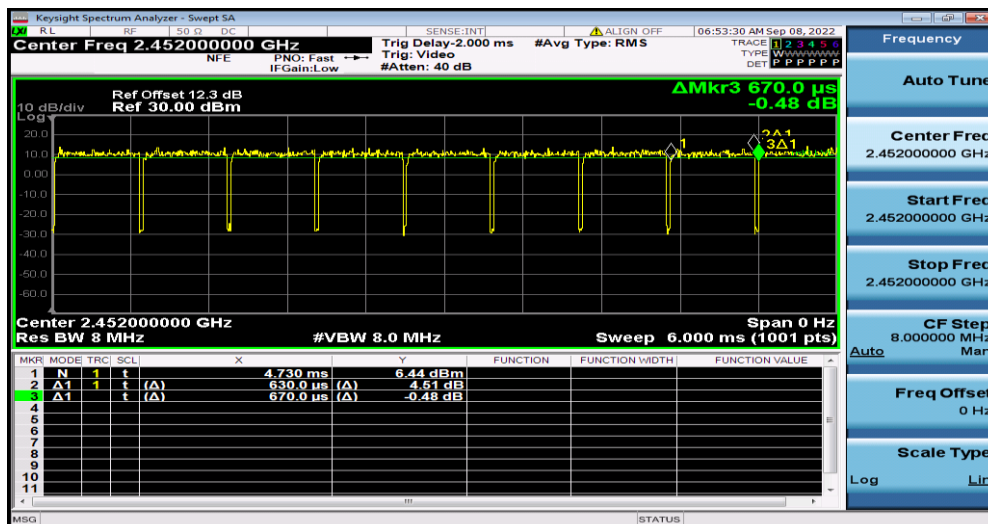
11N40MIMO_Ant1_2452
