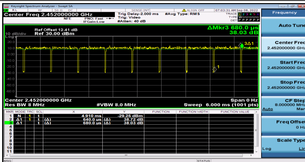
11N40MIMO_Ant2_2452
