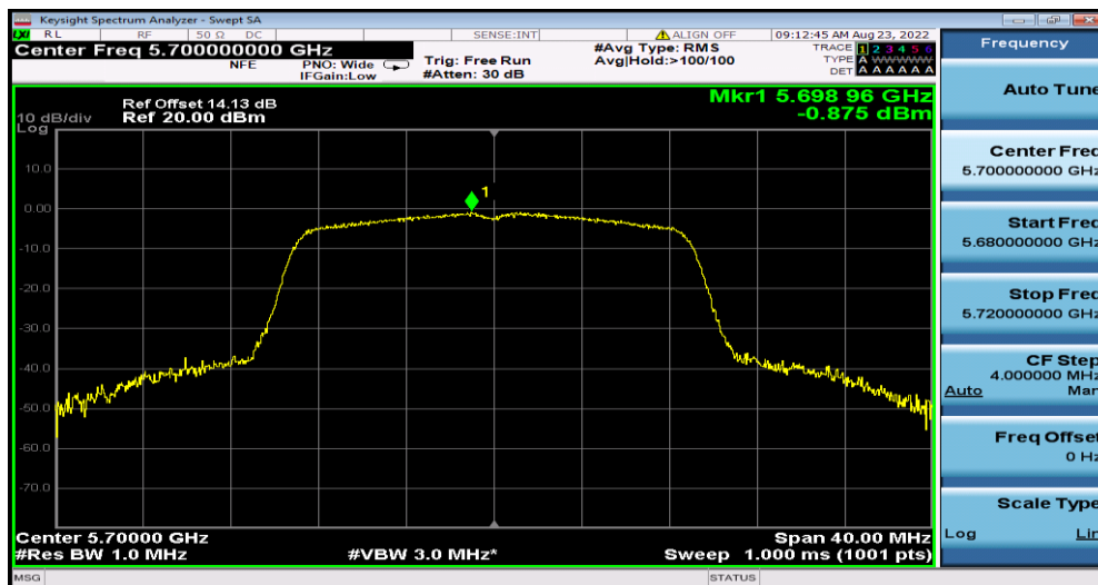
11N20MIMO_Ant1_5700
