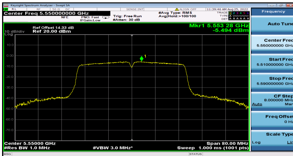
11N40MIMO_Ant1_5550
