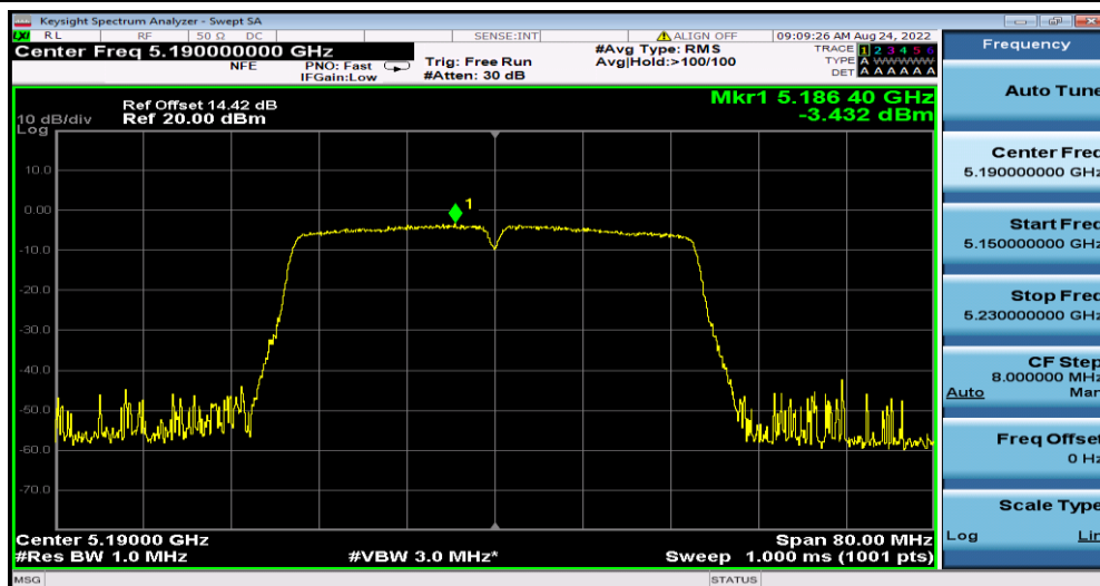
11N40MIMO_Ant1_5190
