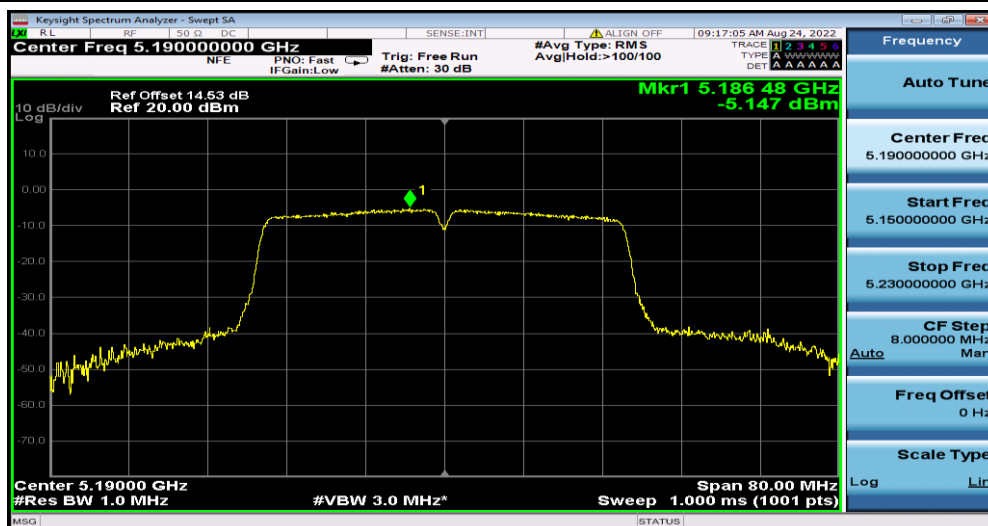
11N40MIMO_Ant2_5190
