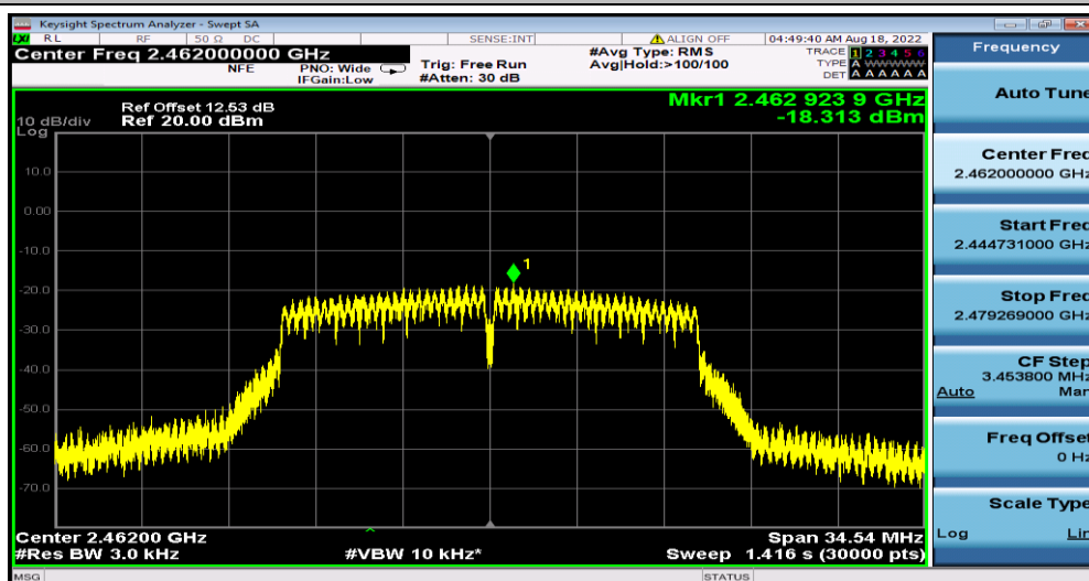
11G_Ant2_2462
