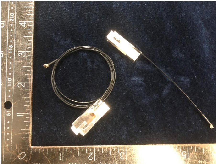
Optional antenna
