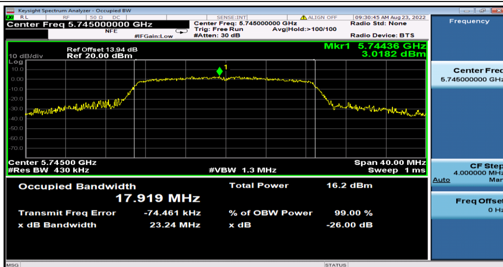
11N20MIMO_Ant1_5745
