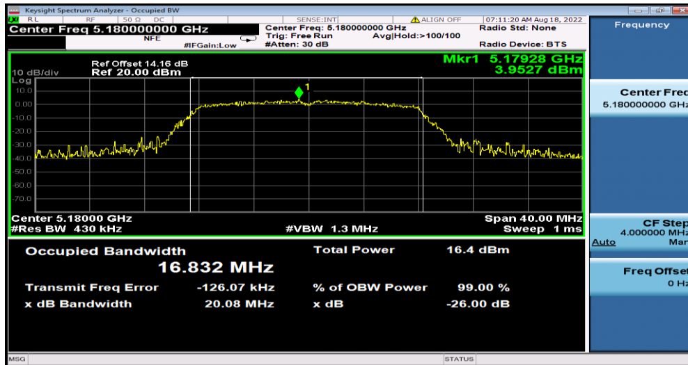
11A_Ant1_5180
